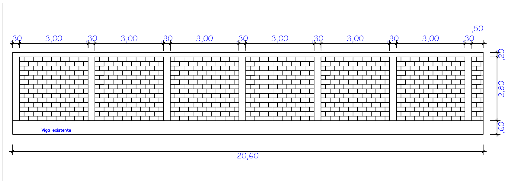
Vista do muro Escala 1:100
